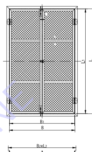
C型-方角双扇钢丝网门 TYPE C- WIRE MESH DOUBLE DOOR
