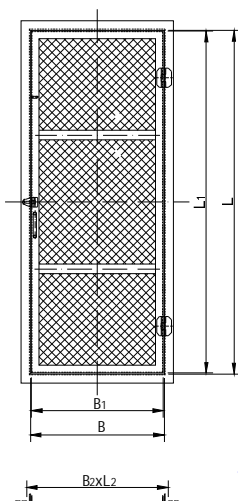
B型-方角单扇钢丝网门 TYPE B-SINGLE WIRE MESH DOOR
