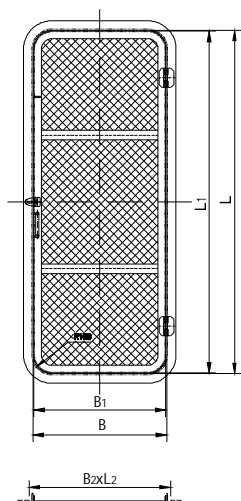
A型-圆角单扇钢丝网门 TYPE A-SINGLE WIRE MESH DOOR(ROUND CORNER)
